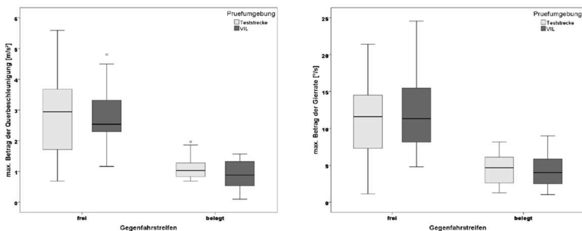
Abbildung 7: maximale Beträge der Querbeschleunigung (links) und der Gierrate (rechts)
